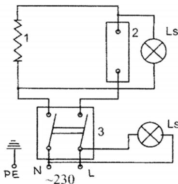
Rys. 3. Schematy elektryczne ogrzewaczy.
