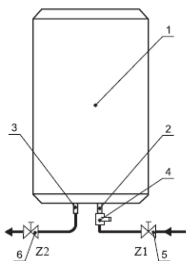
Rys.2 Schemat podłączenia ogrzewaczy do sieci wodociągowej.
